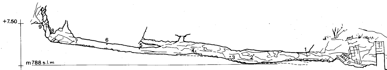
SEZIONE LONGITUDINALE
